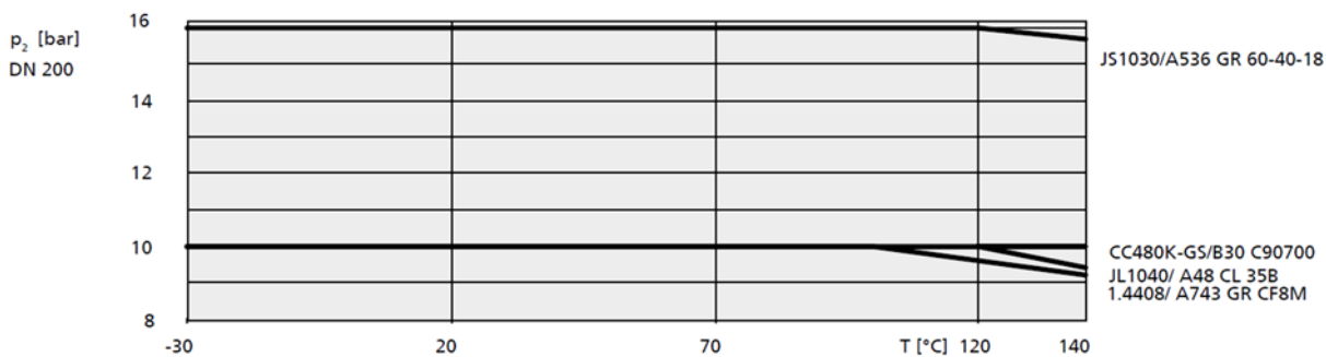
图. 2: 泵的压力和温度限值 DN 200
