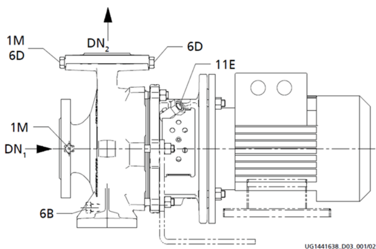
图. 5: 外冲洗A型泵盖单机械密封（FA）
