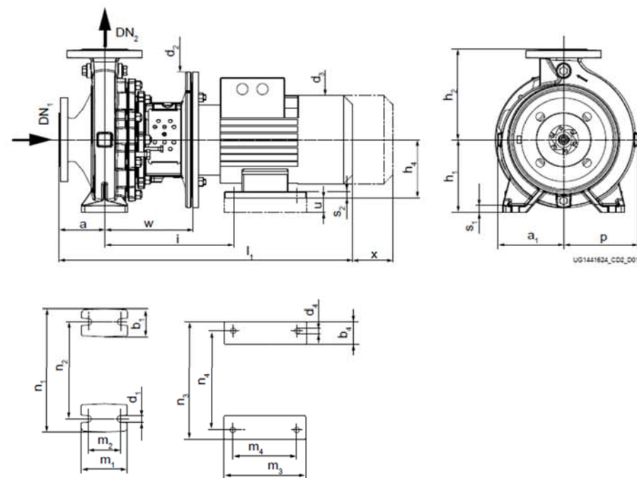
带支撑脚和电机脚的泵组（电机尺寸132至180）
