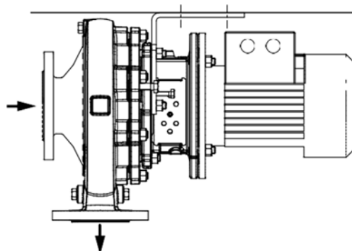
图. 16: 卧式安装，上方固定，泵组带支撑脚，电机尺寸 \leq 112
