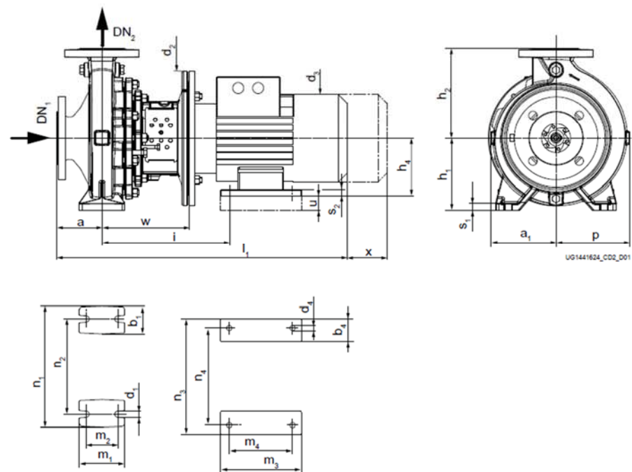
带支撑脚和电机脚的泵组（motor sizes 132 to 180）
