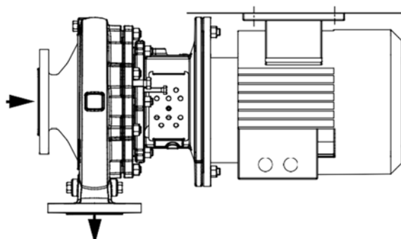
图. 17: 卧式安装，上方固定，泵组，电机尺寸 132 - 180
