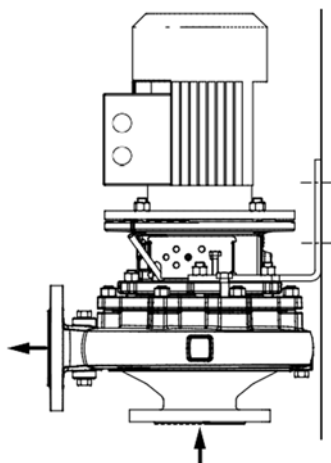
图. 18: 立式安装，泵组带支撑脚，电机尺寸 \leq 112
