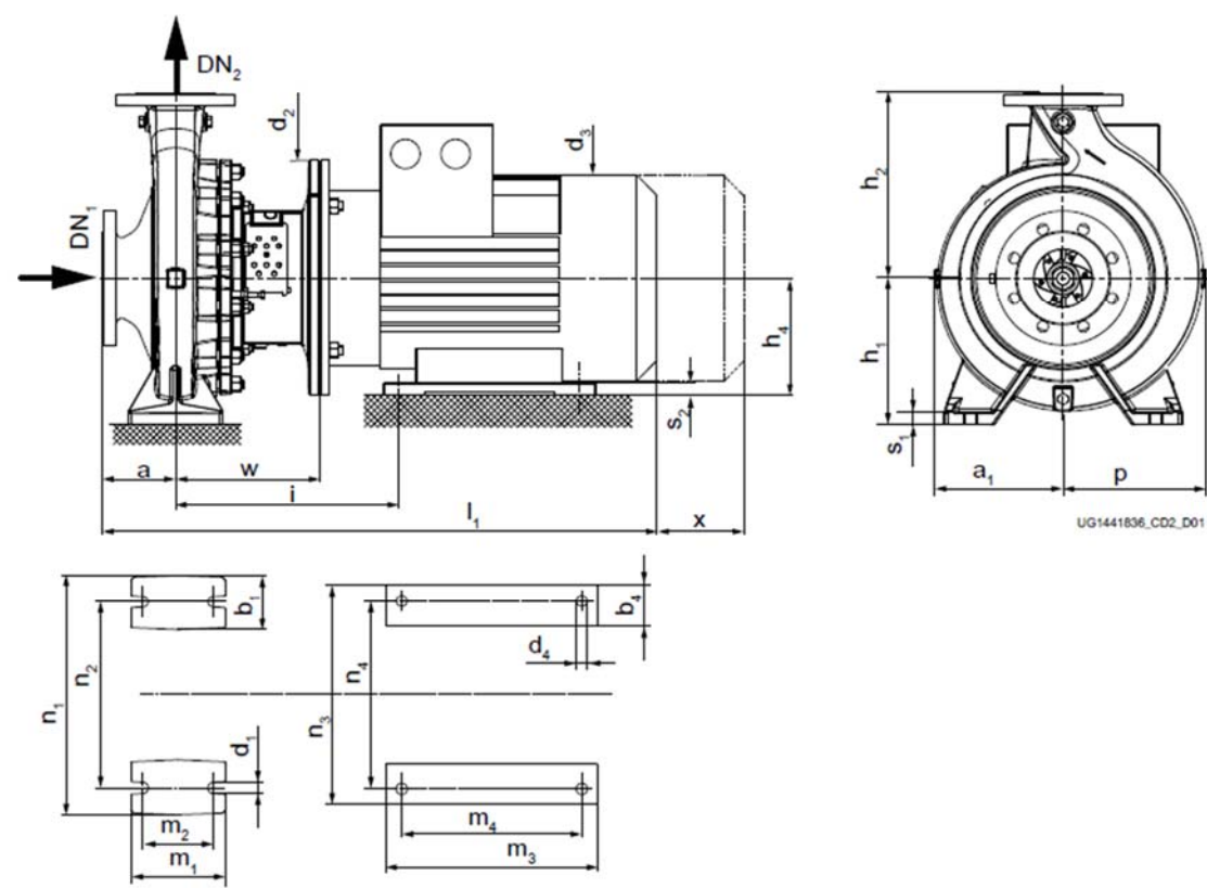
带支撑脚和电机脚的泵组（电机尺寸200至315，4级）
