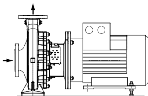
图. 15: 卧式安装，下方固定，泵组带支撑脚，电机尺寸 200 - 315, 4级
