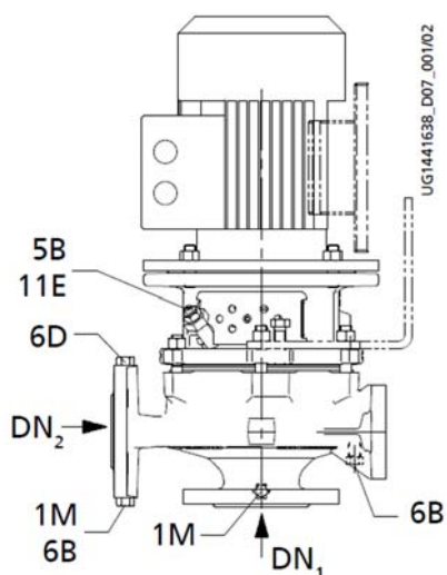
图. 6: A型泵盖的单机械密封, 如果立式安装, 则具有外冲洗 (FA) 和排气功能
