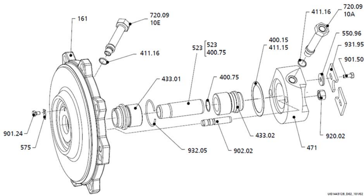
图. 25: 带双机械密封背对背安装的版本
