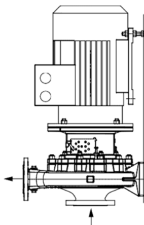
图. 20: 立式安装，泵组带泵壳脚，电机尺寸 200 - 315,
