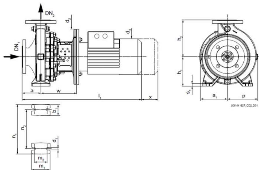
带支撑脚和电机脚的泵组（固定速度版本）， \leq 22 \text{ kW} , n = 2900 \text{ rpm} / 3500 \text{ rpm}
