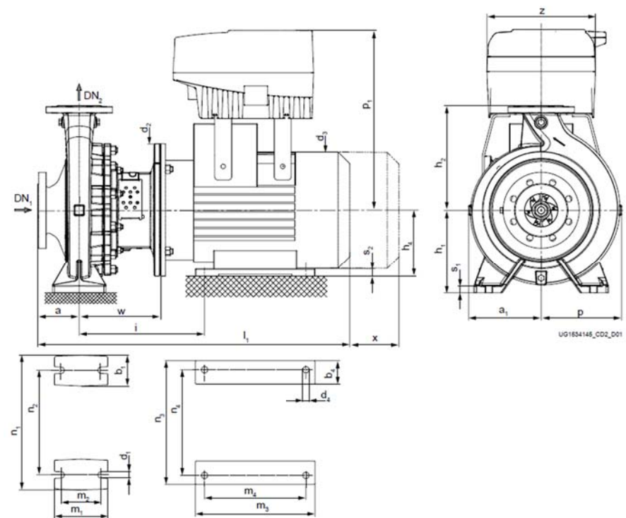
Etabloc PumpDrive (电机尺寸200至225)
