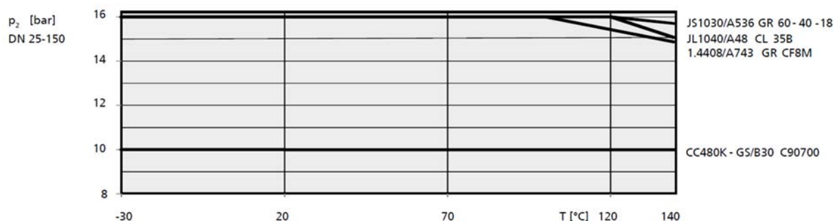
图. 1: 泵的压力和温度限值 DN 25 - DN 150
