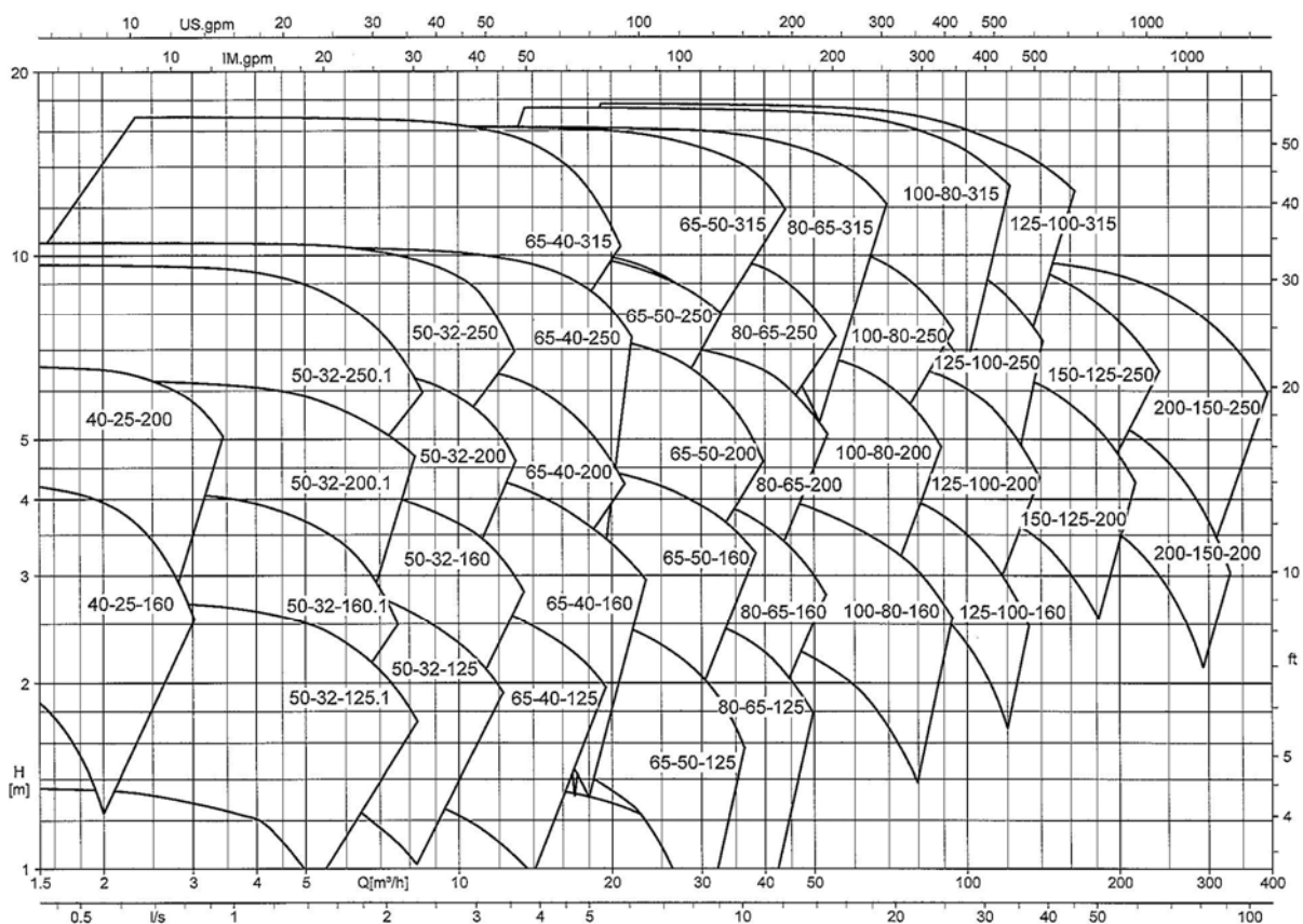
Etabloc, n = 3500 rpm (固定速度版本)
