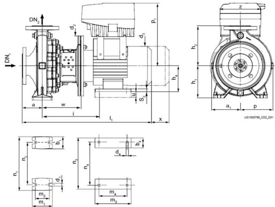
Etabloc PumpDrive (电机尺寸132至180)
