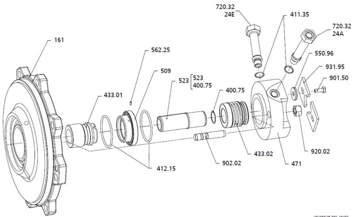
图. 26: 带双机械密封串联安装的版本
