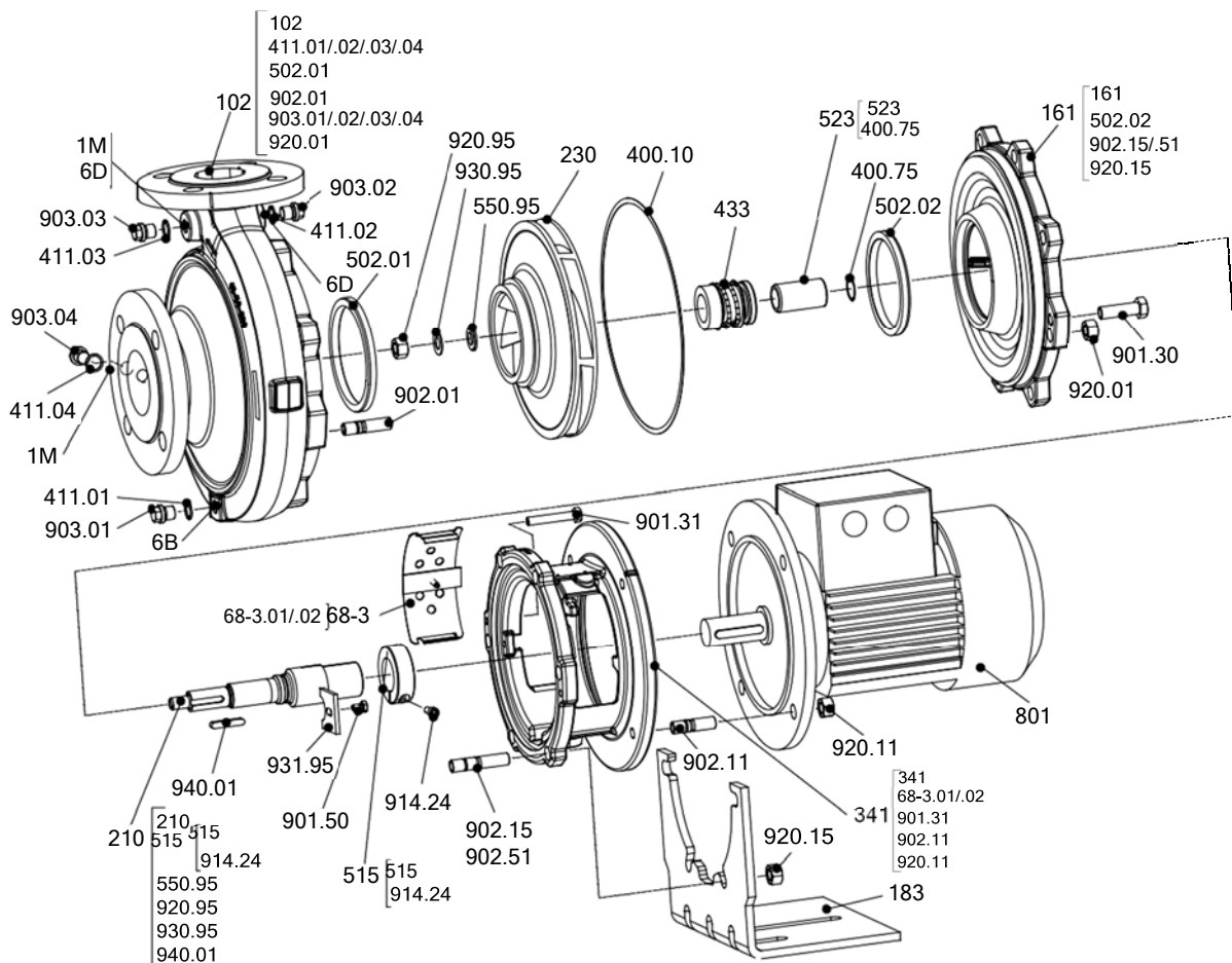
图. 21: 带有单机械密封和螺栓连接泵盖的版本，无泵脚
