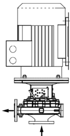
图. 19: 立式安装，泵组带泵壳脚，电机尺寸 132 – 180
