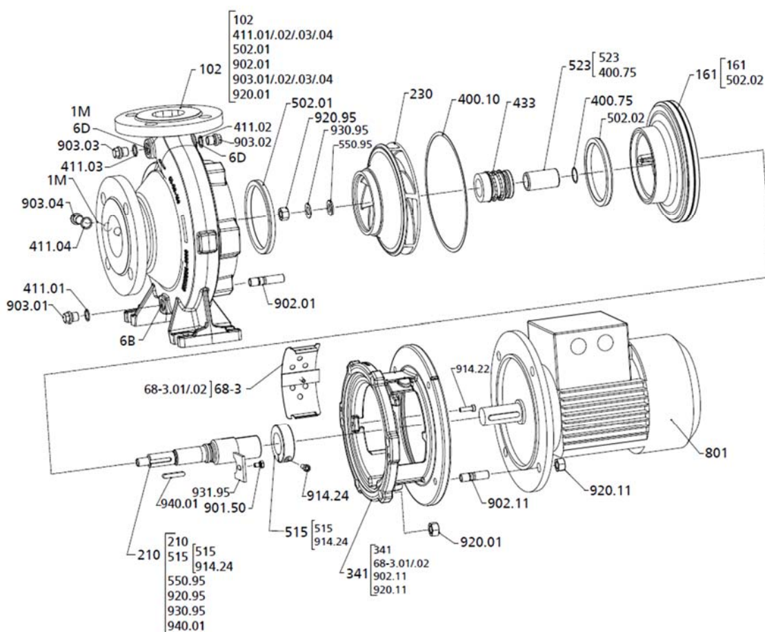
图. 24:带单机械密封和压紧式泵盖的泵组, 有泵脚
