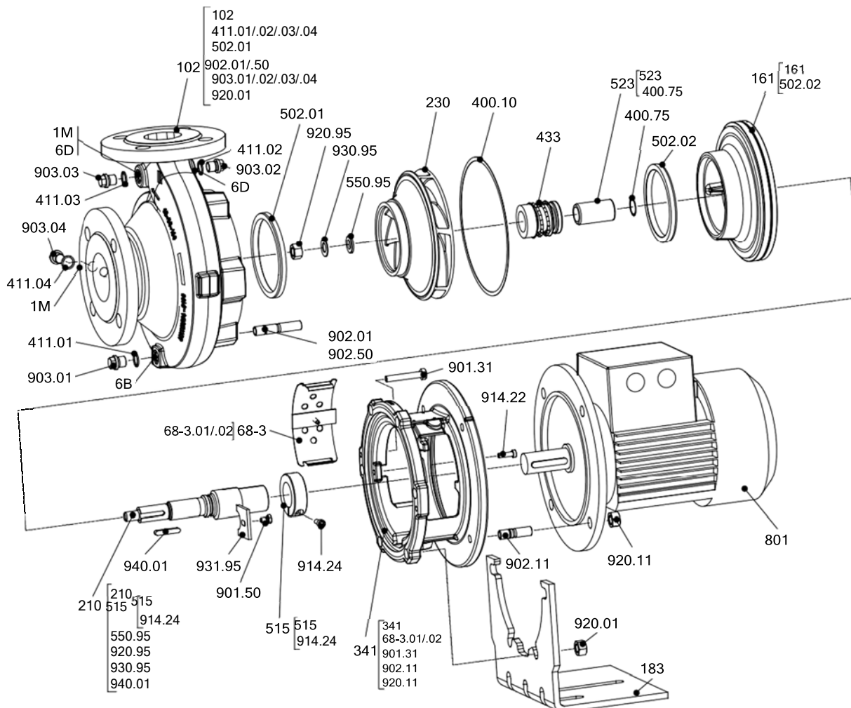
图. 23: 带单机械密封和压紧式泵盖的泵组，无泵脚
