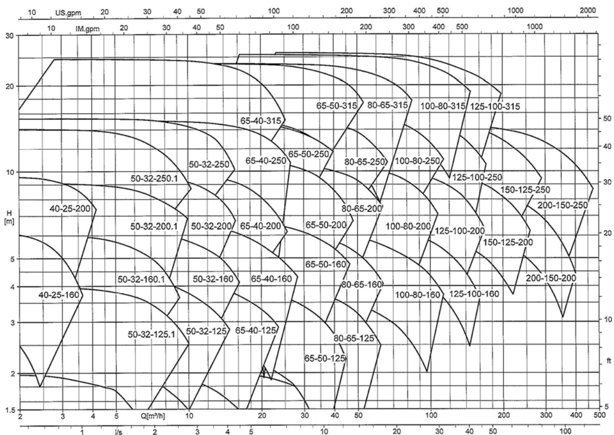
Etabloc, n = 1160 rpm (固定速度版本)
