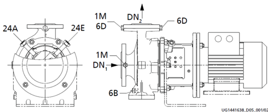
图. 8: 双机械密封串联安装 (TI)
