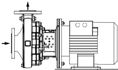
图. 11: 卧式安装，下方固定，泵组，电机尺寸 132 - 180
