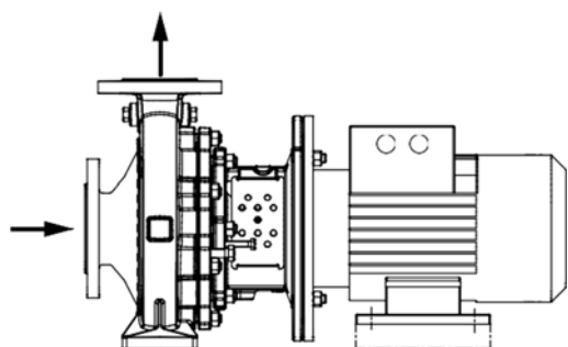
图. 13: 卧式安装，下方固定，泵组带支撑脚，电机尺寸 132 - 180
