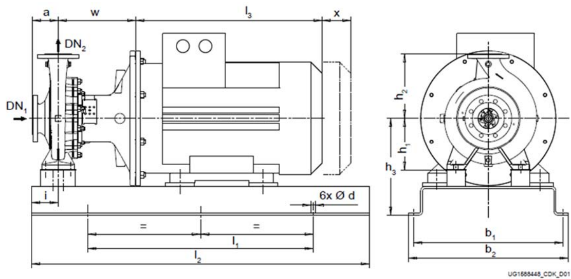
带底座泵组（固定速度版本），55 kW to 110 kW, n = 2900 \text{ rpm} / 3500 \text{ rpm}
