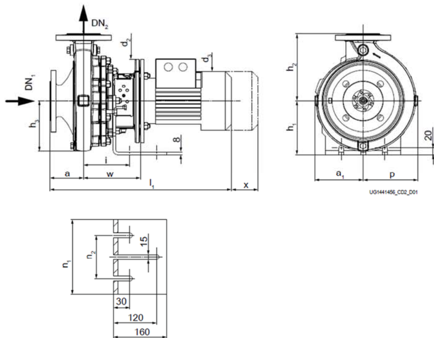
带支撑脚和电机脚的泵组（固定速度版本）， \leq 22 \text{ kW} , n = 1450 \text{ rpm} / 1750 \text{ rpm}
