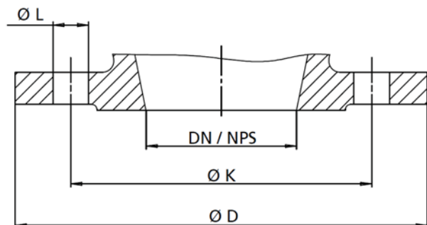
图. 9: 法兰尺寸
