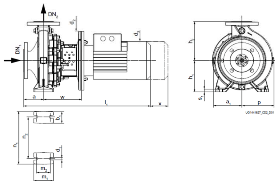
带支撑脚和电机脚的泵组（固定速度版本）， \leq 22 \text{ kW} , n = 1450 \text{ rpm} / 1750 \text{ rpm}
