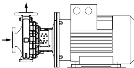
图. 14: 卧式安装，下方固定，泵组，电机尺寸 200 - 315, 2级
