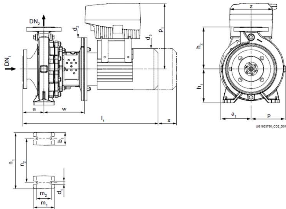
带支撑脚和电机脚的泵组（变速版本）， \leq 22\text{ kW} , n = 2900\text{ rpm} / 3500\text{ rpm}
