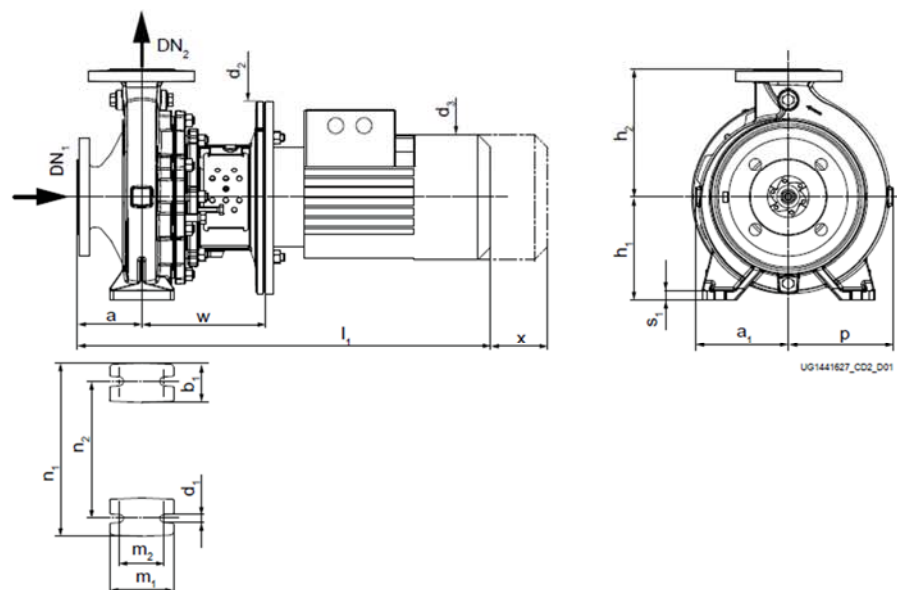
带支撑脚和电机脚的泵组（固定速度版本）， \leq 22 \text{ kW} , n = 960 \text{ rpm} / 1160 \text{ rpm}
