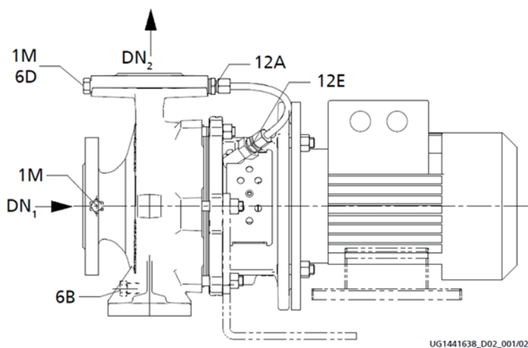
图. 3: A型泵盖单机械密封（AV）和内循环A型泵盖单机械密封（IA）
