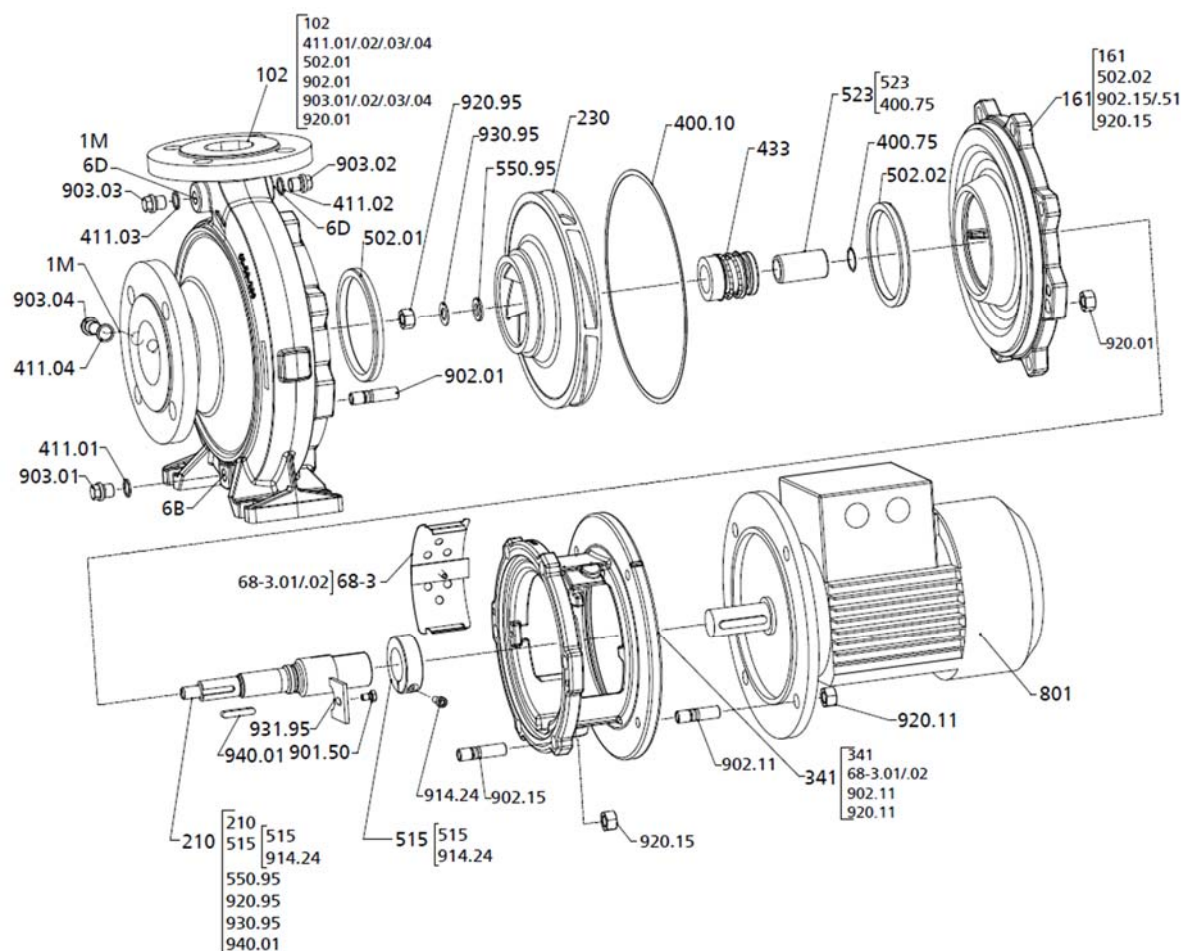
图. 22: 带有单机械密封和螺栓连接泵盖的版本，有泵脚 部件清单 100)
