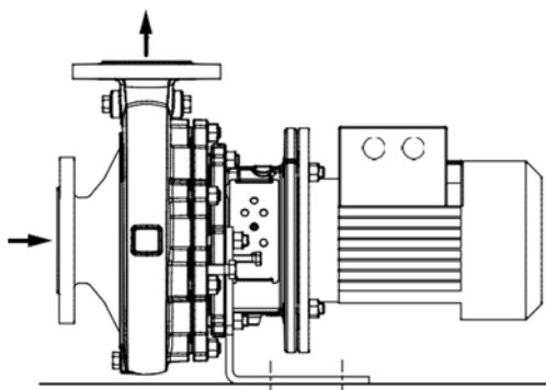
图. 10: 卧式安装，下方固定，泵组带支撑脚，电机尺寸 \leq 112
