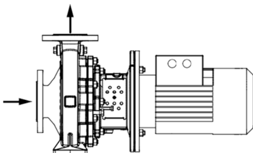
图. 12: 卧式安装，下方固定，泵组带支撑脚，电机尺寸 \leq 112
