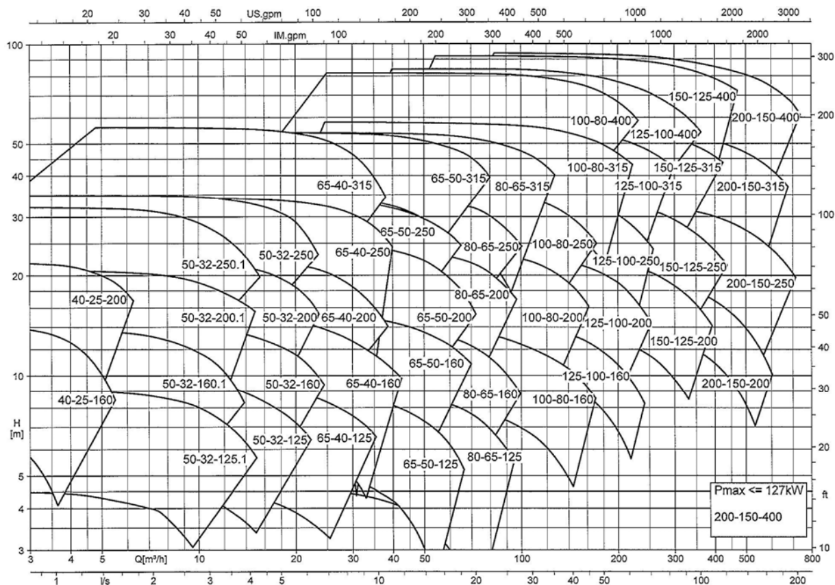
Etabloc, n = 1750 rpm (固定速度版本)
