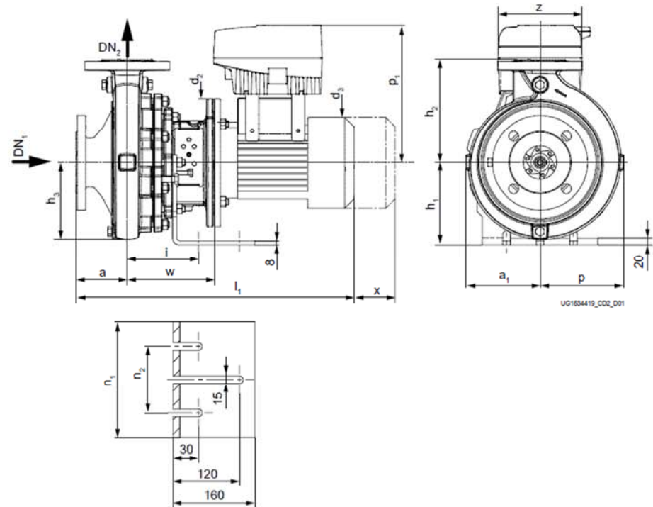
Etabloc PumpDrive（电机尺寸小于 112）
