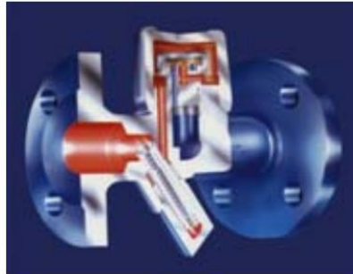
热动力疏水阀 DN15-25 铸钢/高温钢/不锈钢
