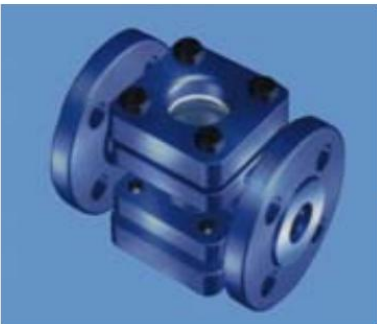
观视镜 DN10-125 PN16-40 铸铁/铸钢/不锈钢
