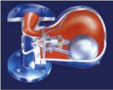
浮球疏水阀 DN15-100, PN16-100 铸铁/球墨铸铁/铸钢/高温钢/不锈钢
